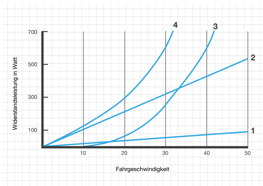
Widerstand beim Radfahren 1 Rollwiderstand 2 Steigungswiderstand (Steigung 5%) 3 Luftwiderstand 4 Gesamtwiderstand
